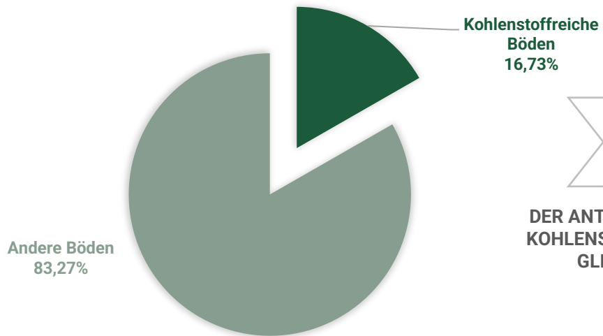
ANTEIL DER KOHLENSTOFFFREICHEN BÖDEN AN DER GESAMTFLÄCHE DER STADT CUXHAVEN
