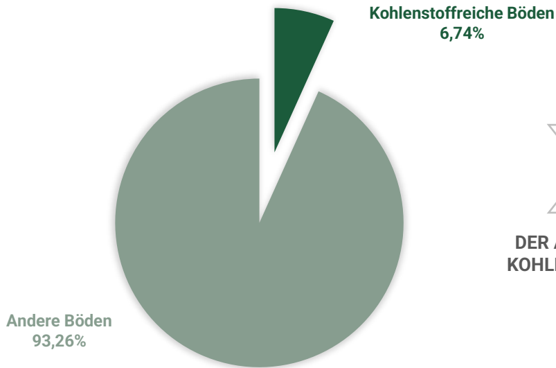
ANTEIL DER KOHLENSTOFFFREICHEN BÖDEN AN DER GESAMTFLÄCHE DER EG WURSTER NORDSEEKÜSTE
